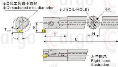
进给方向 Feed direction
