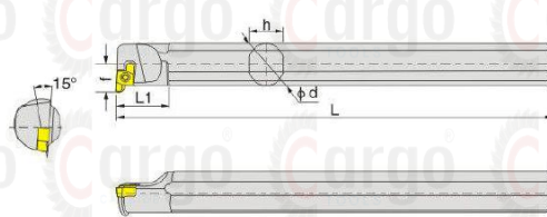
内径槽刀 Internal diameter groove cutter
